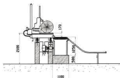
SEZ. C-C
